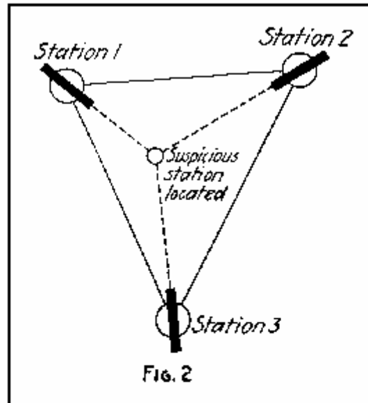
Tres estaciones receptoras formando un triángulo ajustarán sus indicadores de dirección a la máxima intensidad de señal e inmediatamente se localizará la estación sospechosa
