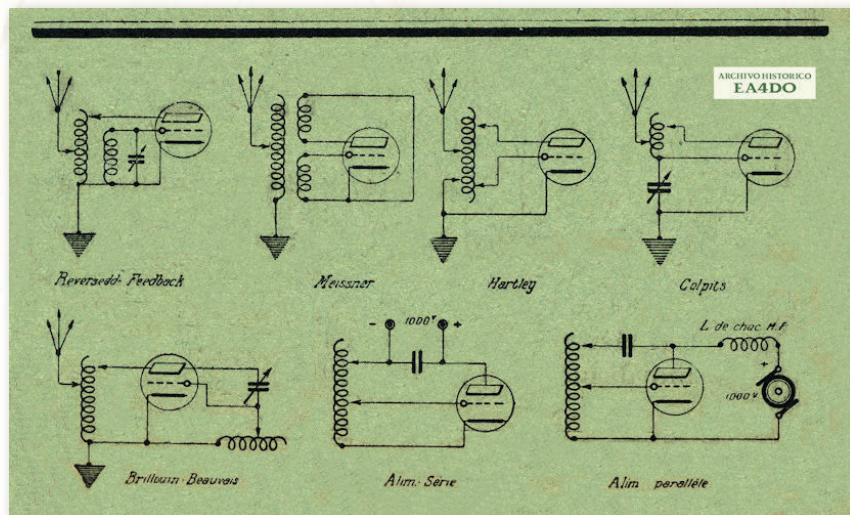
Habituales circuitos de emisión publicados en 1925 por Journal des 8 y experimentados por Enrique Ricart, EA3AN, previamente a la concesión del indicativo EAR-73. (Colección EA1AB/EAR-18)
